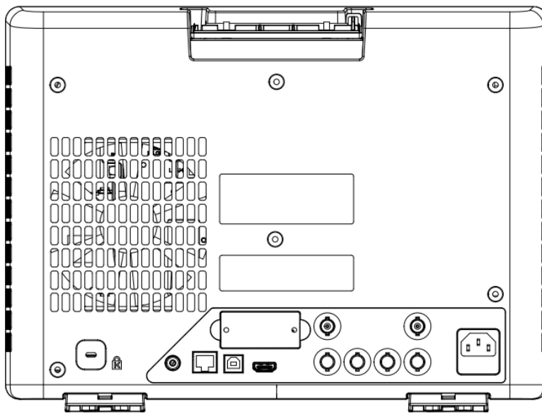
图 5-2 背视图
