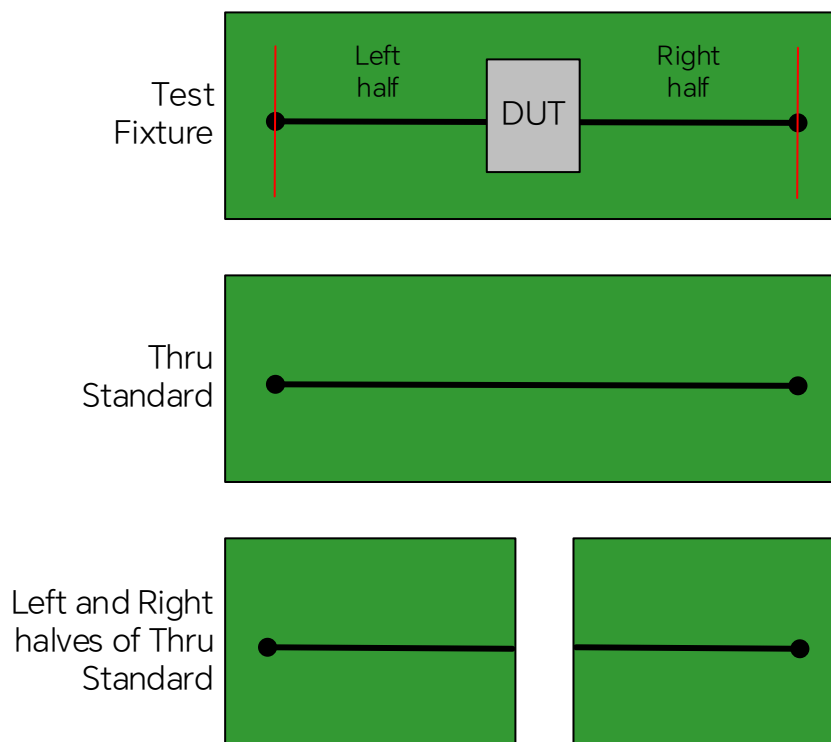
图 14-1 单端口夹具
