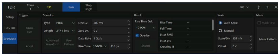
图 10-13 眼图选项卡
