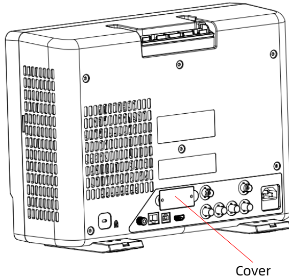
图 5-7 OCXO 选件安装步骤
