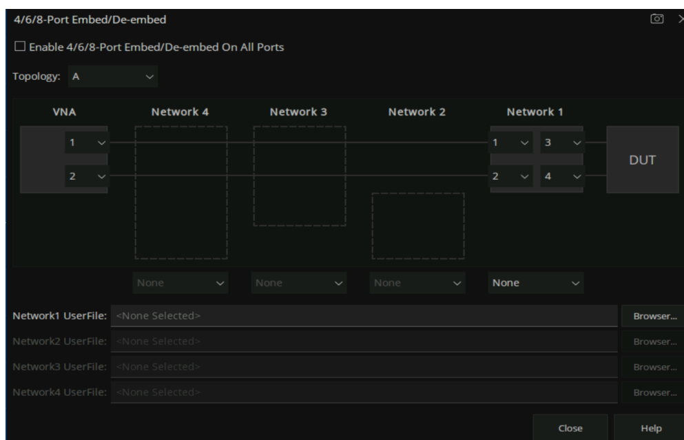
图 7-11 去嵌入界面
