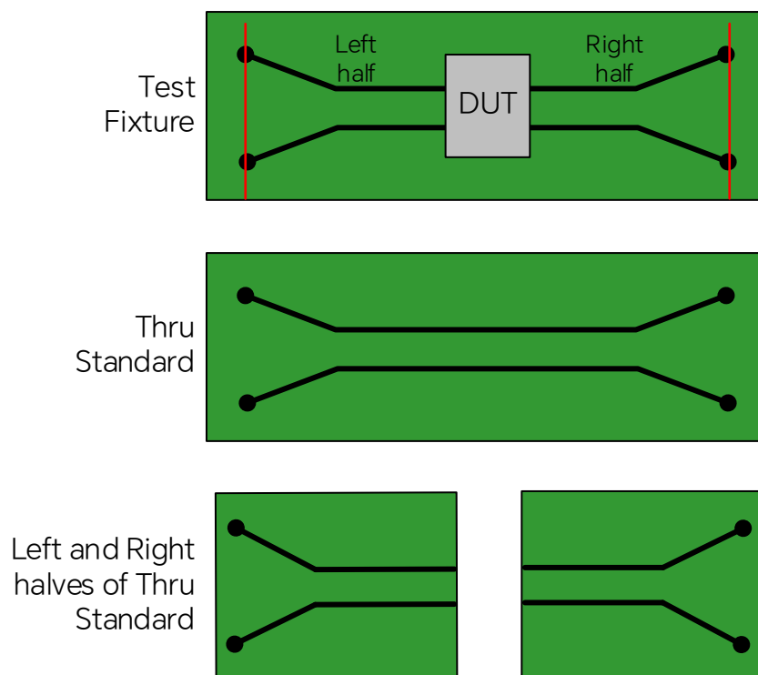
图 14-2 差分夹具
