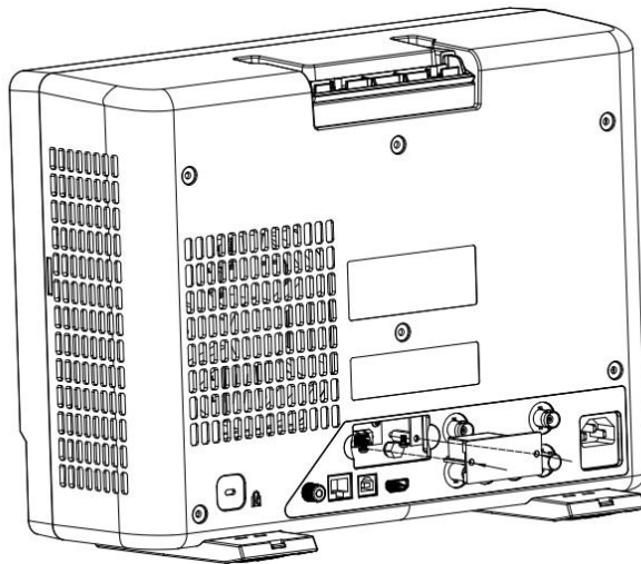
图 5-8 OCXO 选件安装步骤
