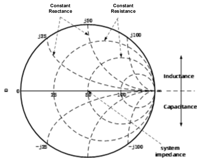
图 6-6 史密斯圆图示意图
