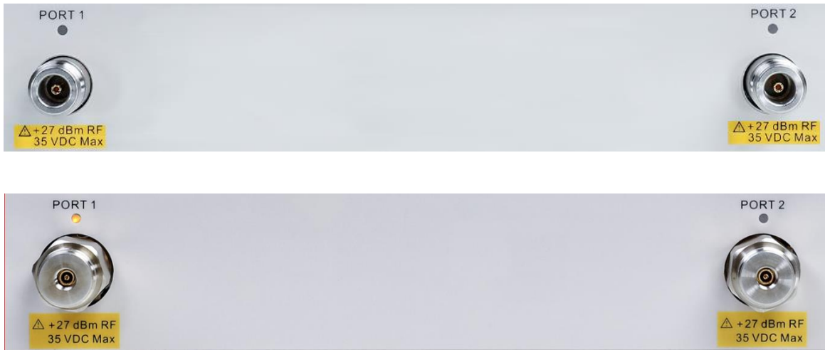
图 5-5 前面板上射频连接器（2 端口网络分析仪）
