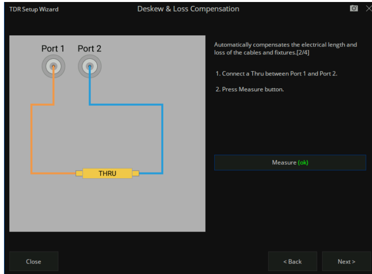
图 10-5 TDR 延时损耗补偿校准向导
