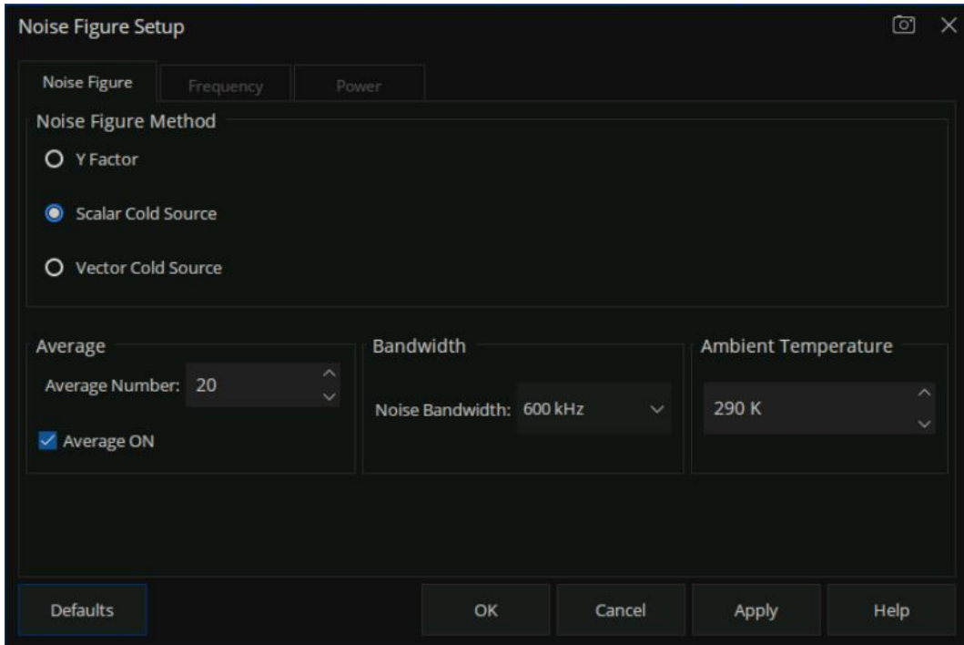
图 18-19 噪声系数法为标量冷源法
