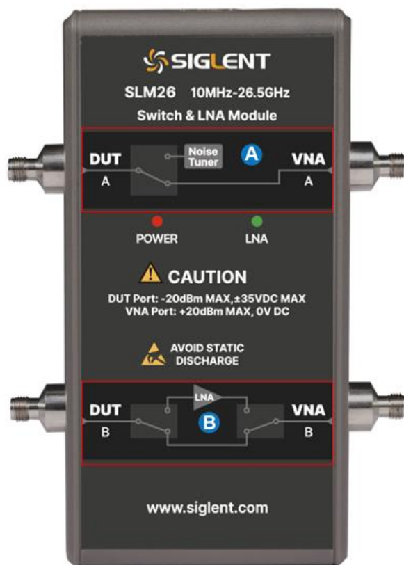
图 18-2 SLM 系列开关和低噪放模块
