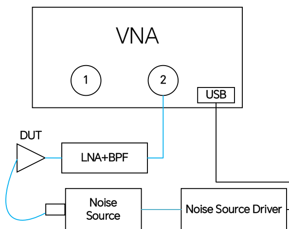
图 18-7 Y 因子法测量原理图
