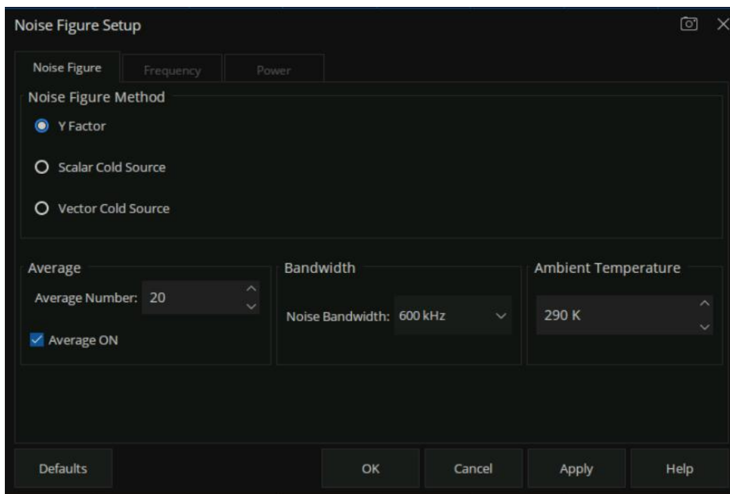
图 18-8 噪声系数法为 Y 因子
