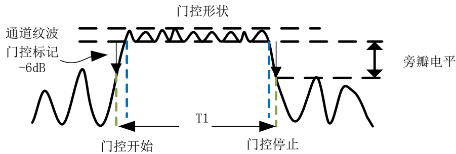
图 8-15 门控示意图
