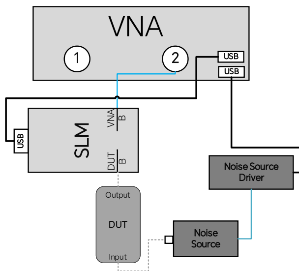
图 18-14 Y 因子测量连接示意图
