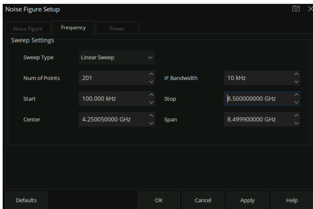
图 18-4 Frequency 选项卡
