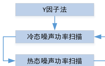
图 18-6 Y 因子法测量扫描流程
