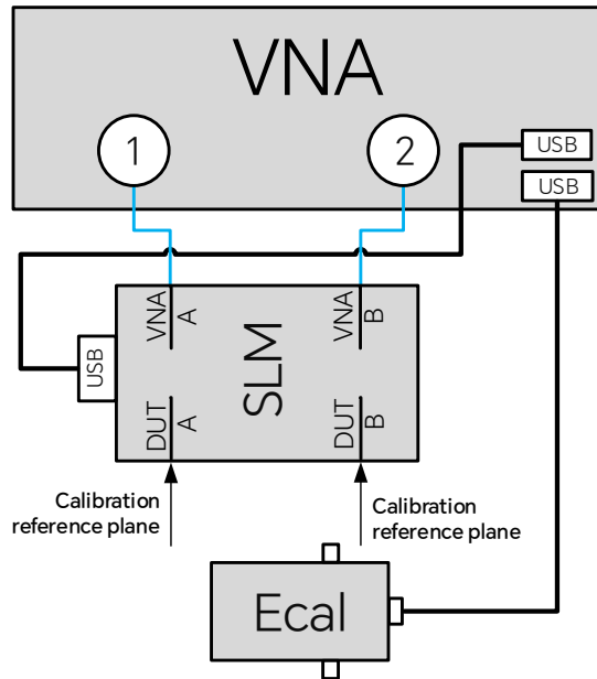
图 18-25 冷源法电子校准连接图
