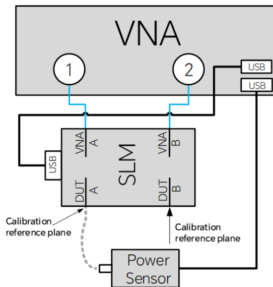
图 18-28 冷源法功率计连接图
