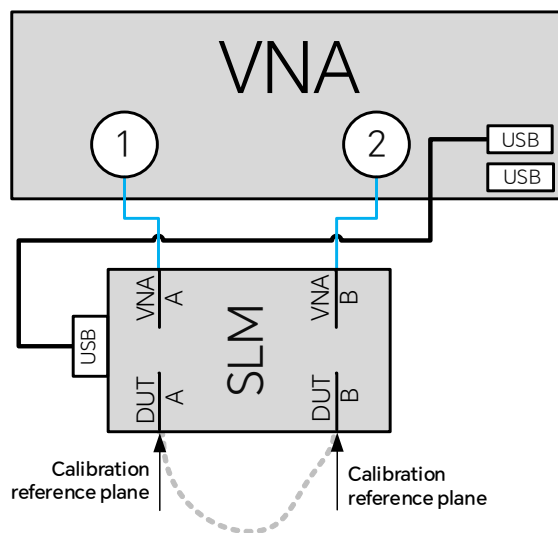
图 18-30 冷源法噪声接收机校准连接图
