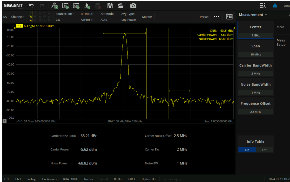
图 11-17 载噪比测量界面
