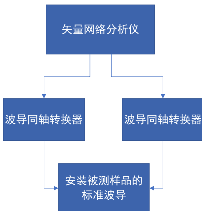
图 15-1 测试原理图
