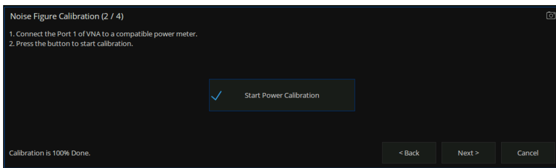
图 18-29 冷源法功率校准向导界面
