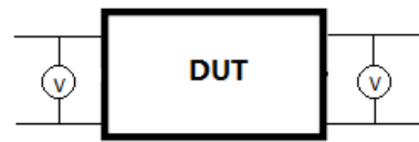
Fig2.2 平衡设备
