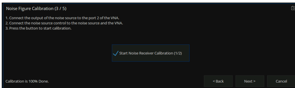
图 18-34 冷源法噪声源校准向导界面
