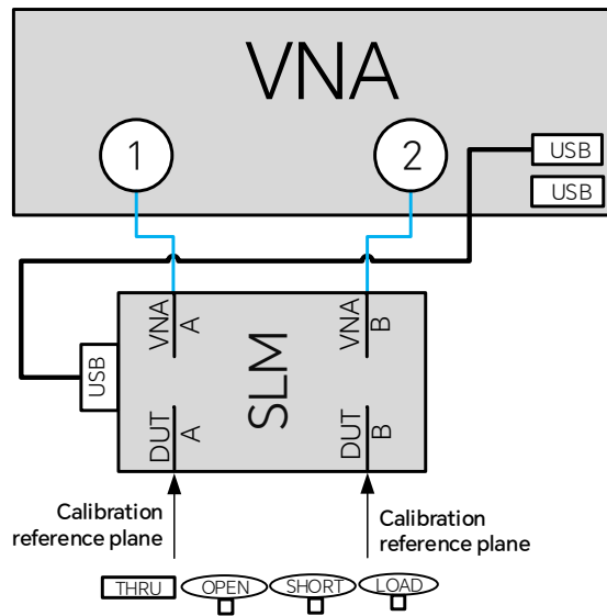
图 18-22 冷源法机械校准连接图
