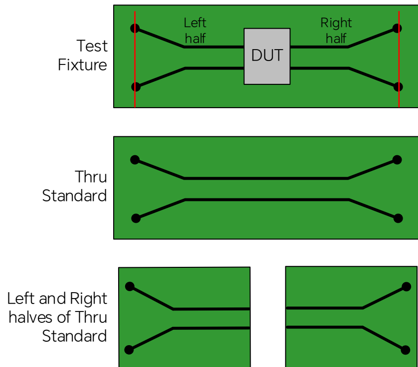
图 19-2 差分夹具
