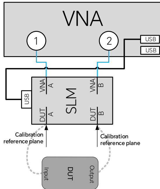
图 18-40 冷源法测量连接示意图
