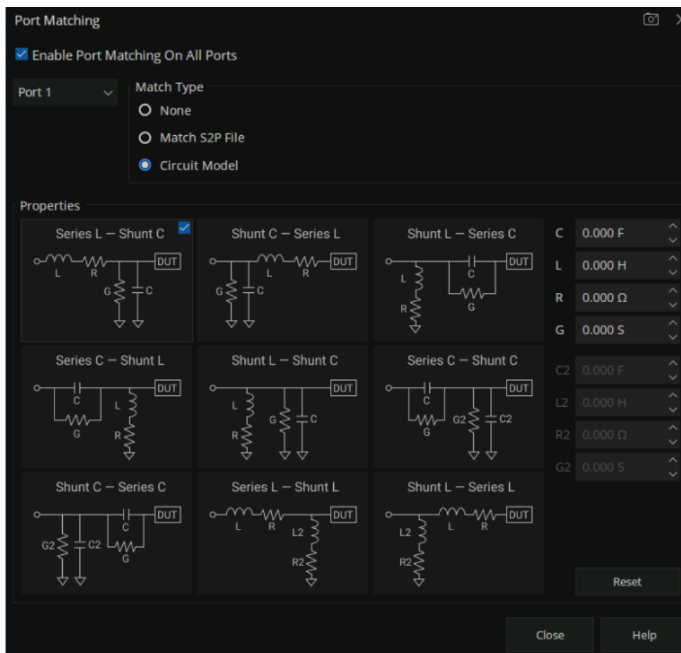
图 7-8 端口匹配
