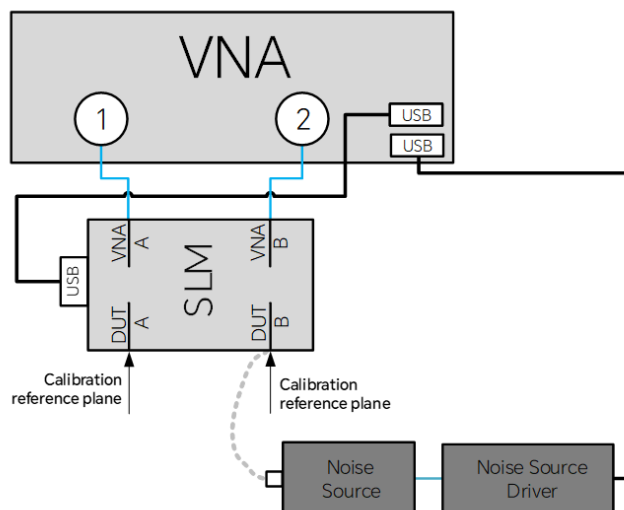
图 18-33 冷源法噪声源连接图
