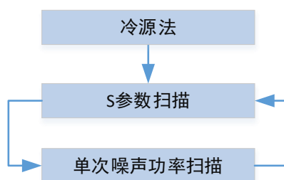
图 18-15 标量冷源法测量扫描流程
