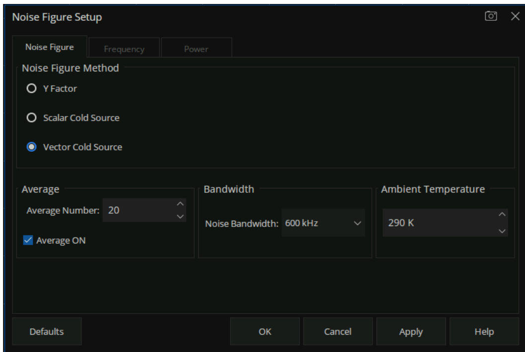
图 18-3 Noise Figure 选项卡
