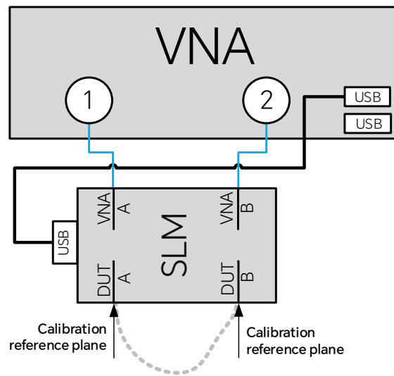
图 18-37 噪声带宽校准连接图
