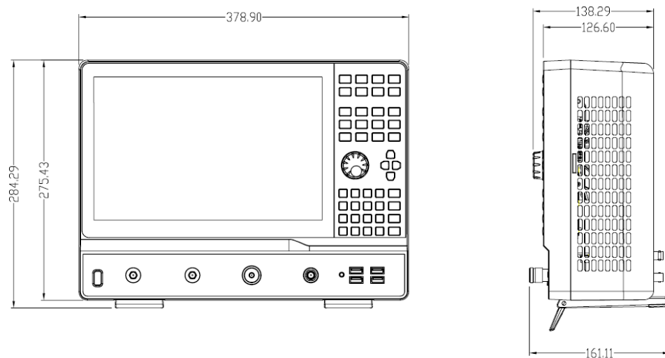
图 5-1 前视图和侧视图
