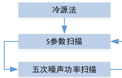
图 18-17 矢量冷源法测量扫描流程
