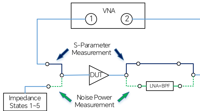
图 18-18 矢量冷源法测量原理图
