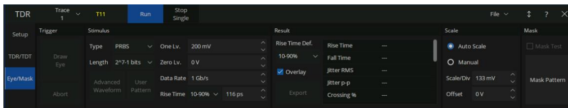
图 10-13 眼图选项卡
