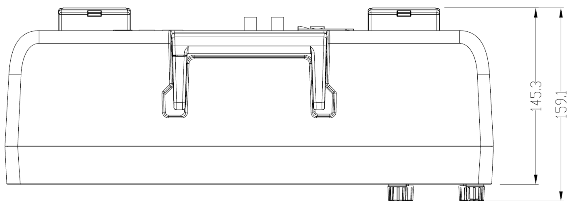
俯视图
