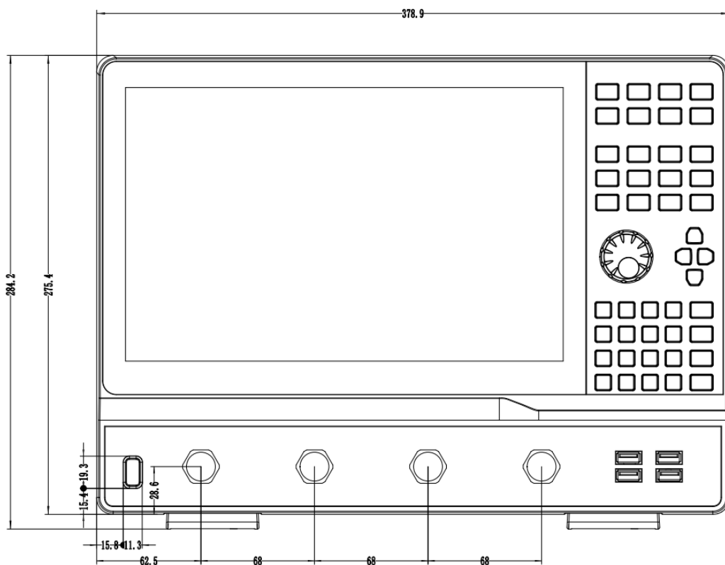
正视图
