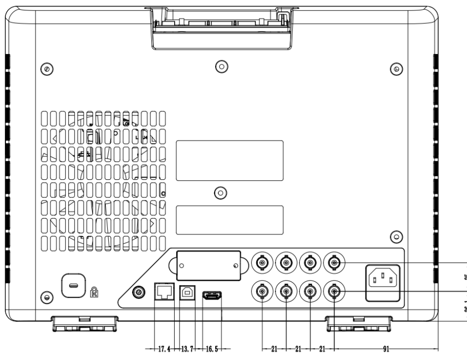
背视图
