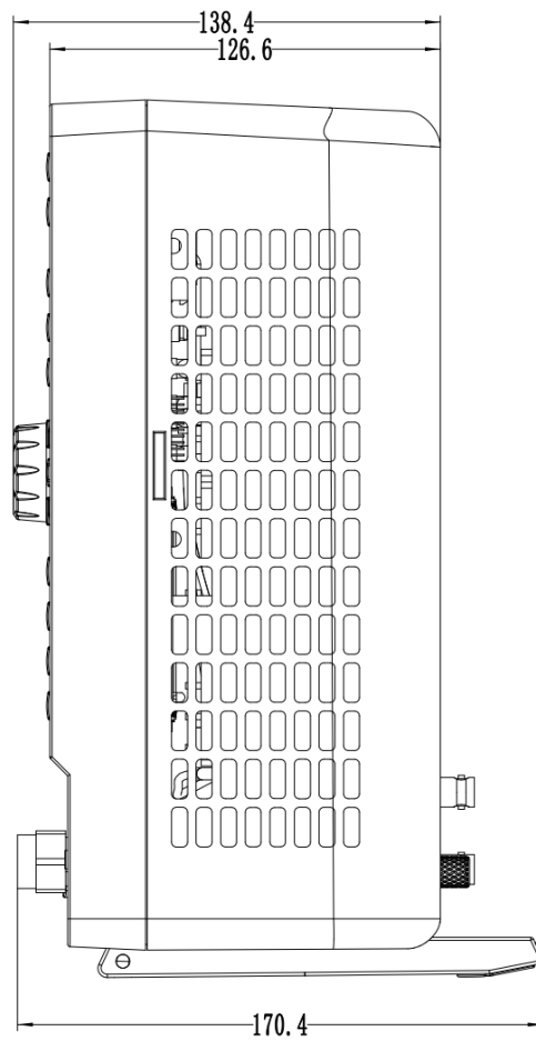
侧视图
