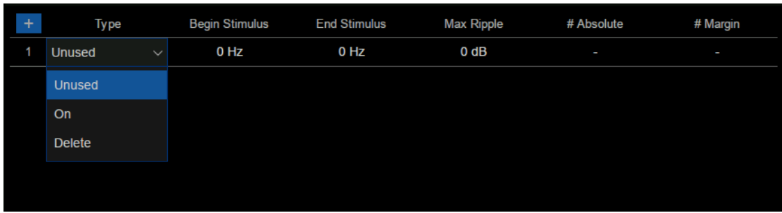
图 8-11 纹波极限线设置界面
