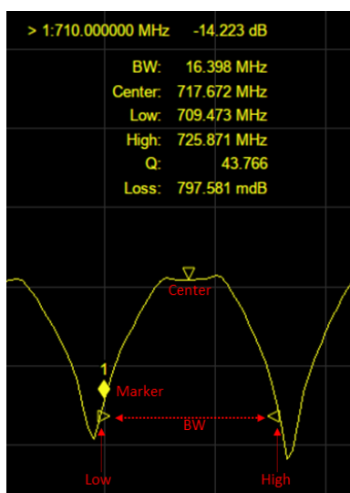
图 8-2 带宽搜索示例
