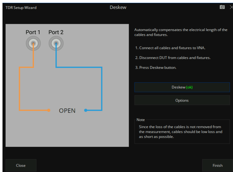
图 10-4 TDR 延时补偿校准向导
