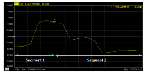
图 6-3 使用 X 轴点间距
