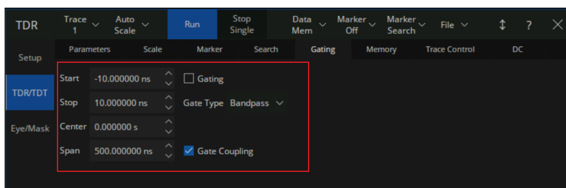
图 10-12 时域门控设置
