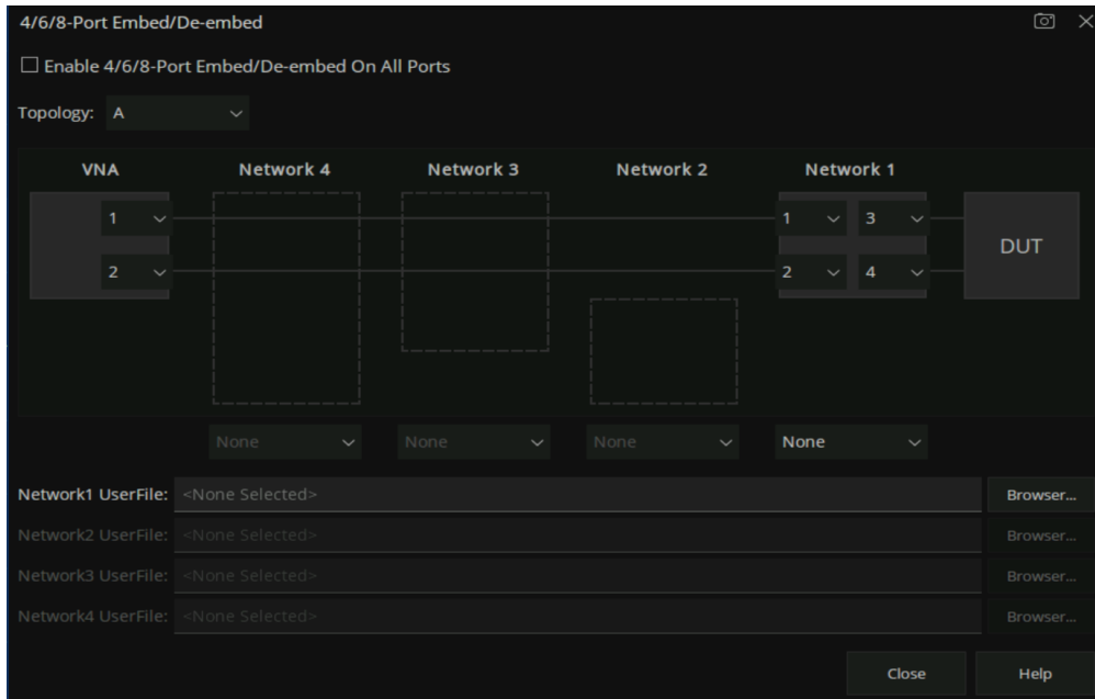
图 7-35 去嵌入界面
