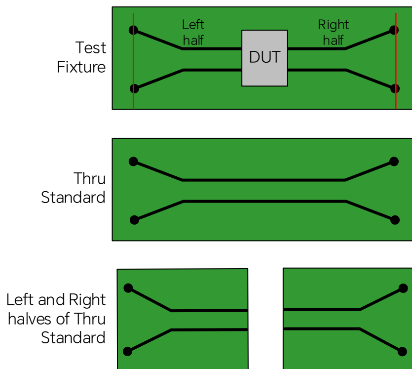
图 15-2 差分夹具
