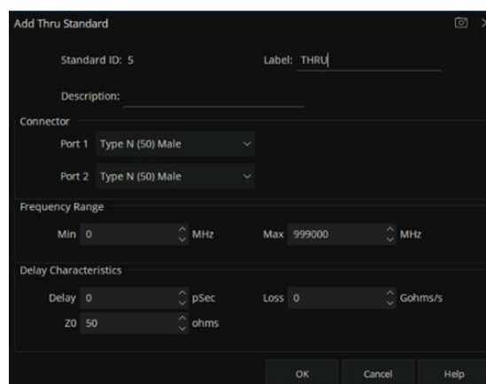
图 7-17 THRU 特性界面
