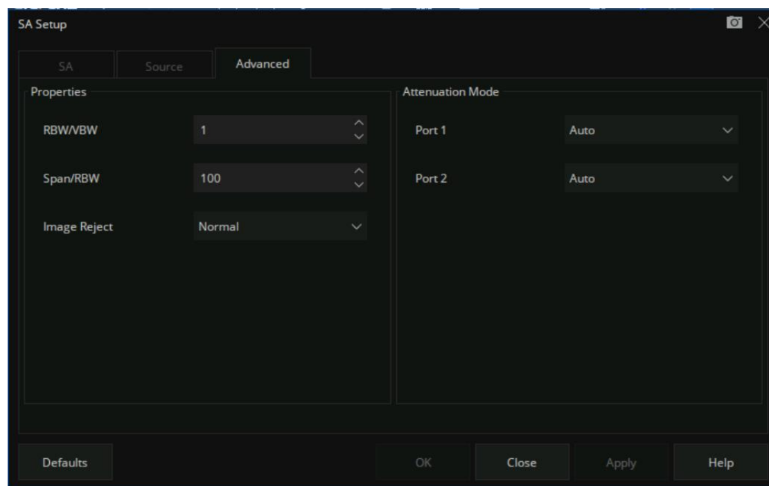
图 11-9 SA Setup 的 Advanced 选项卡界面
