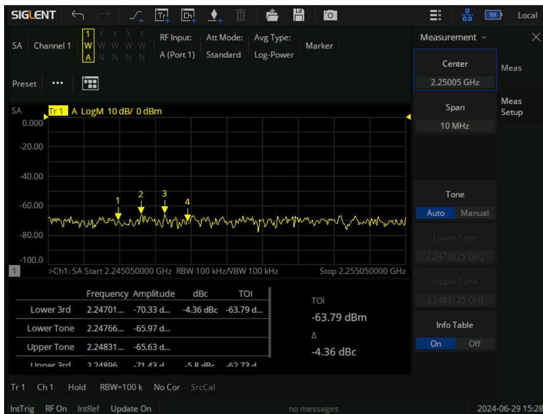
图 11-15 三阶交调测量界面
