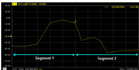
图 6-2 不使用 X 轴点间距
