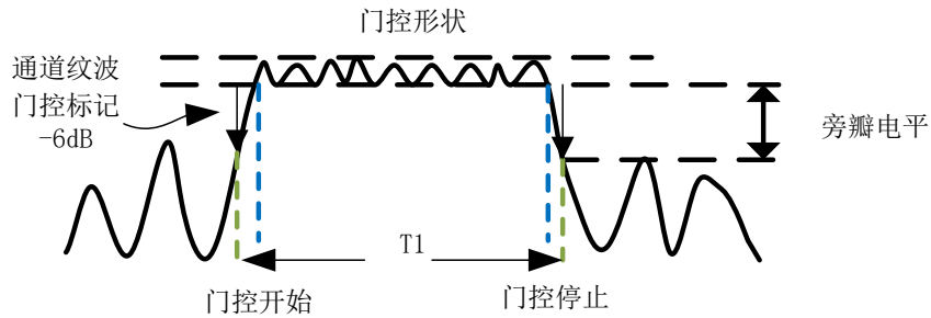
图 8-15 门控示意图
