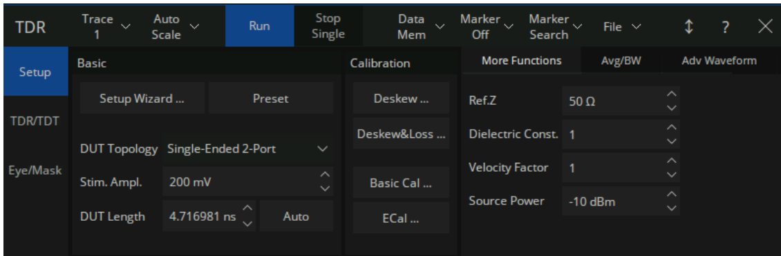
图 10-6 Setup 选项卡
