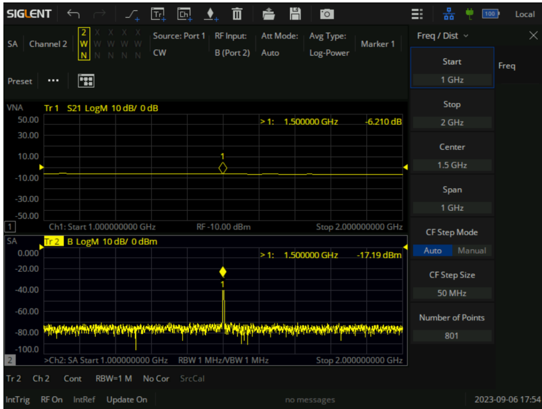
图 11-3 通过按【Freq】键进行 SA 频率相关参数设置
