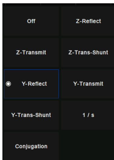
图 8-3 参数转换种类
