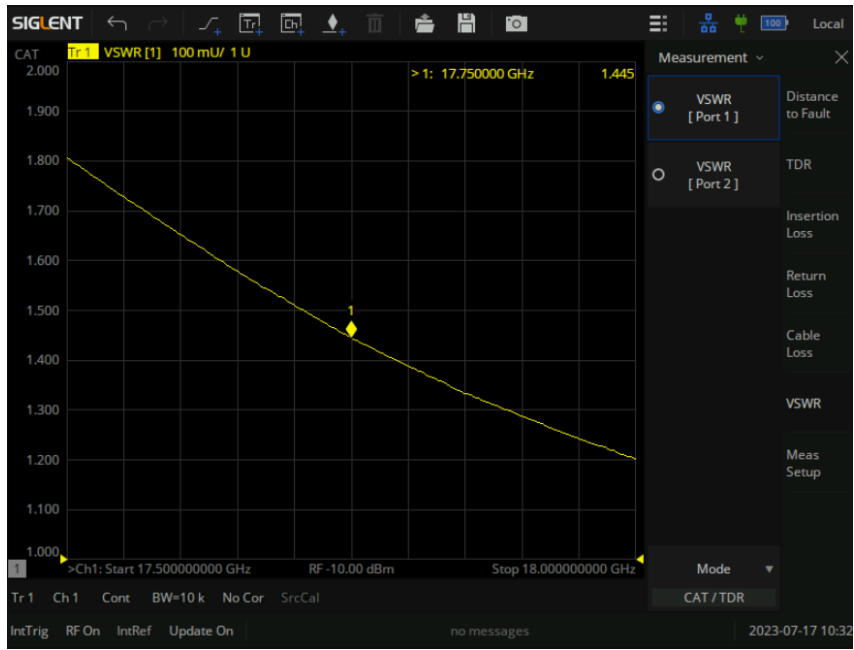
图 13-9 驻波比测量界面
