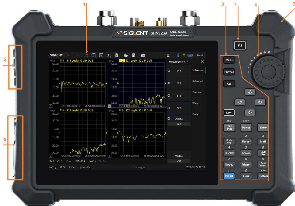
图 5-4 前面板
