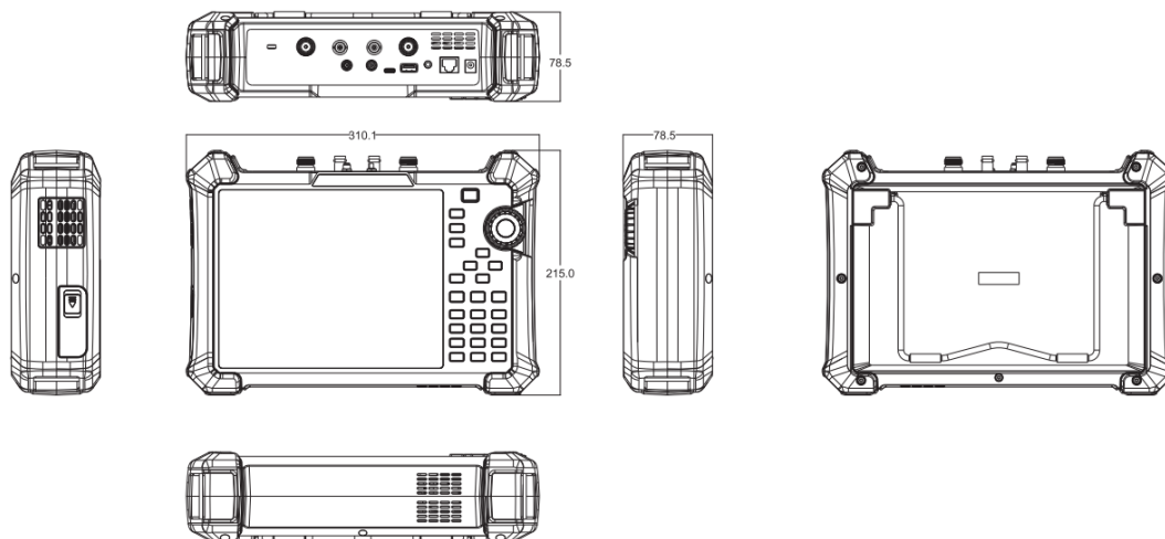
图 5-1 正侧视图
