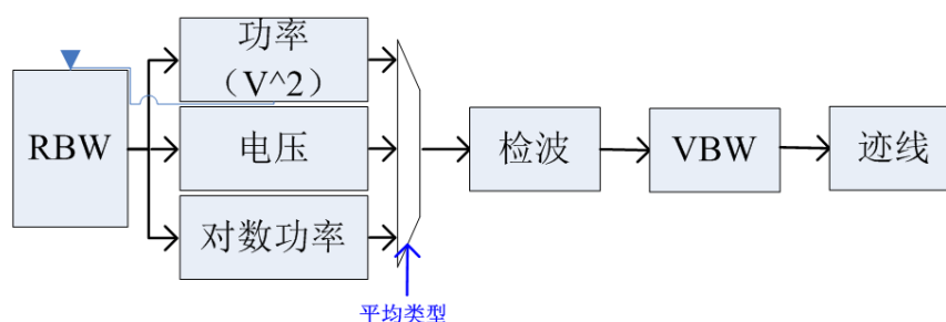
图 2-6 平均类型
