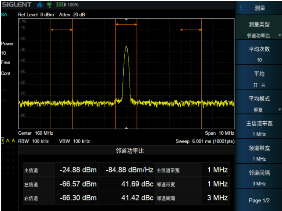
图 2-8 邻道功率比
