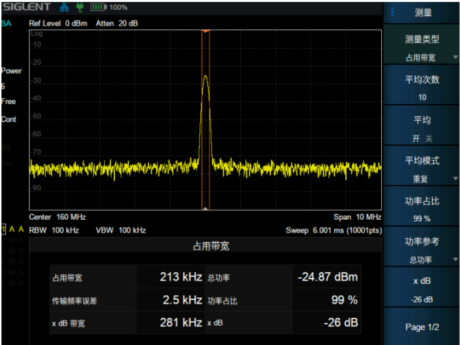
图 2-9 占用带宽
