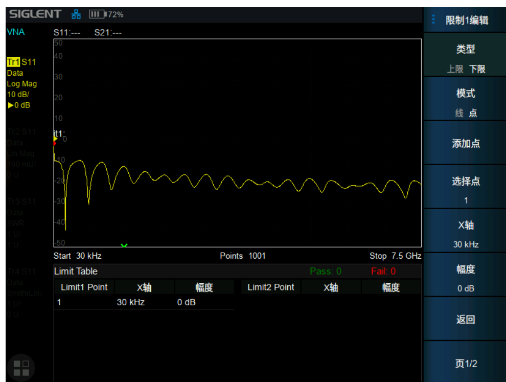
图 4-3 限制编辑
