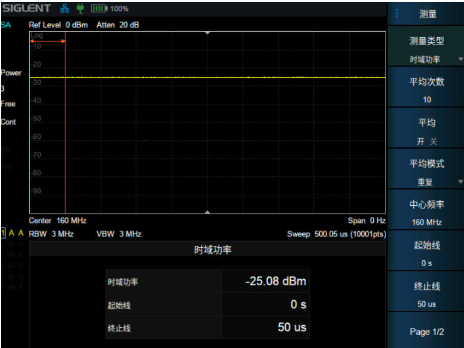
图 2-10 时域功率
