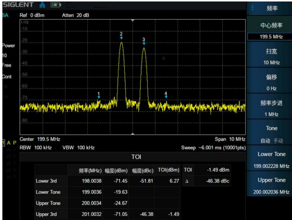
图 2-11 三阶交调
