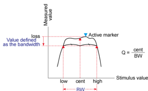
图 4-2 带宽的选择
