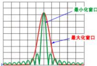
图 3-8 凯瑟窗
