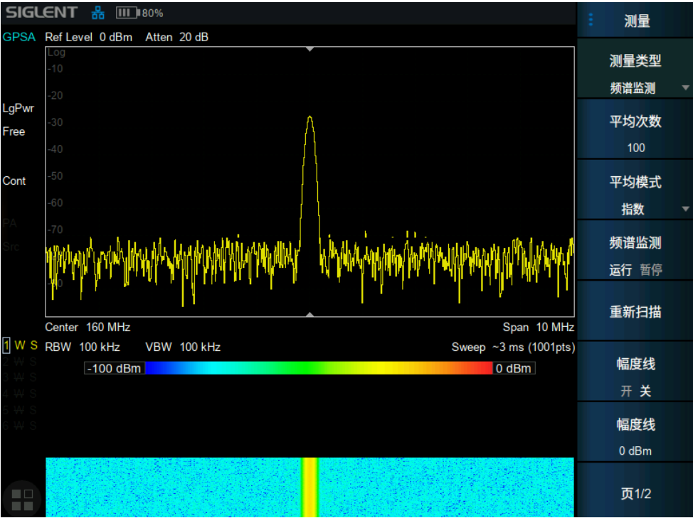
图 2-12 频谱监测
