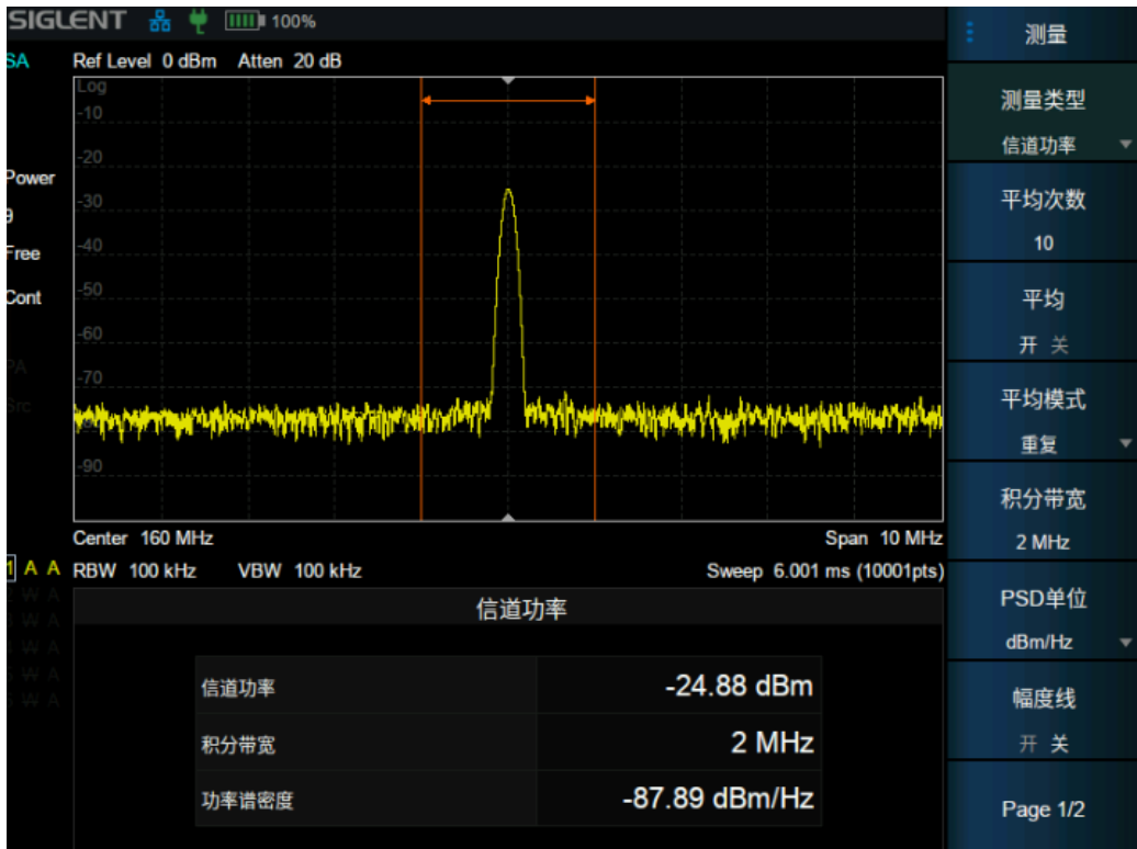
图 2-7 信道功率
