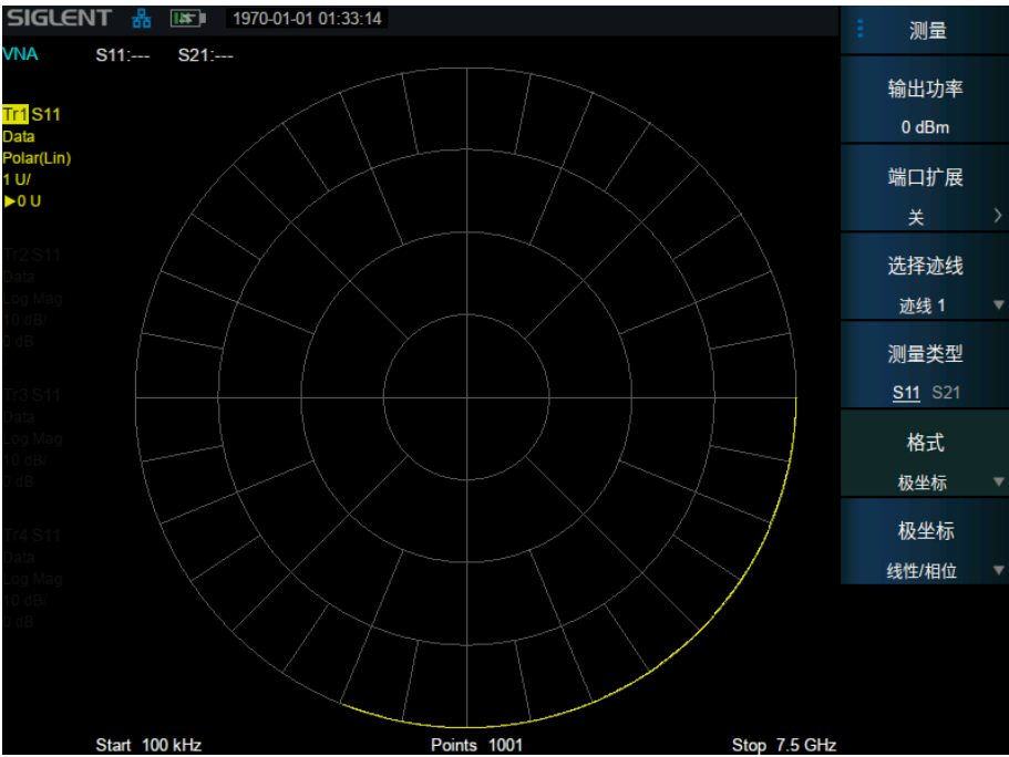
图 4-5 极坐标图
