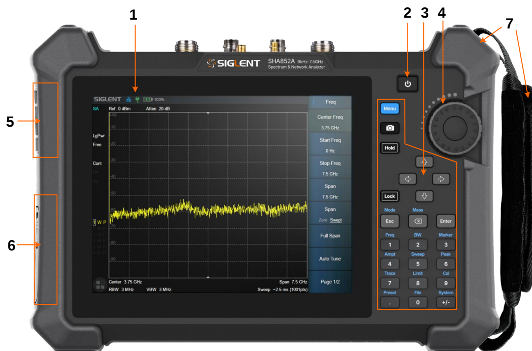
图 1-4 前面板
