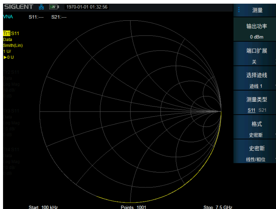
图 4-4 史密斯图
