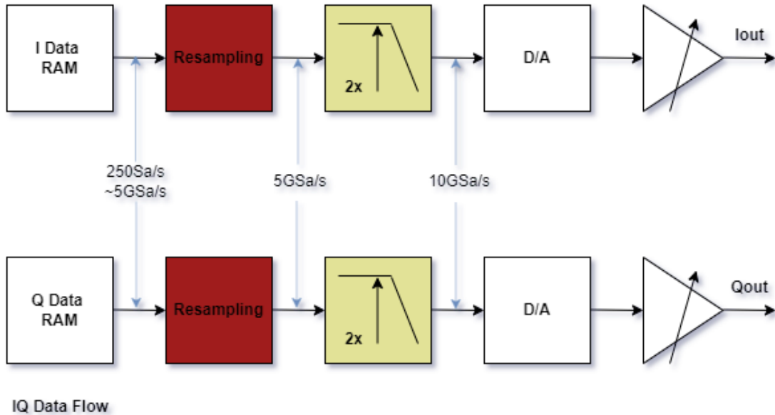
图 13.1 基带 IQ 模式
