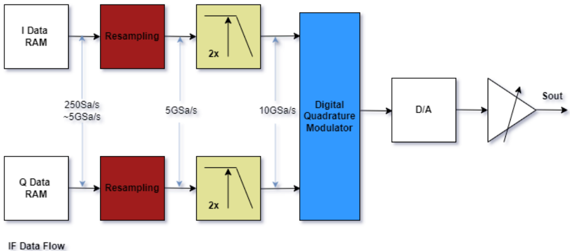
图 13.2 中频信号模式
