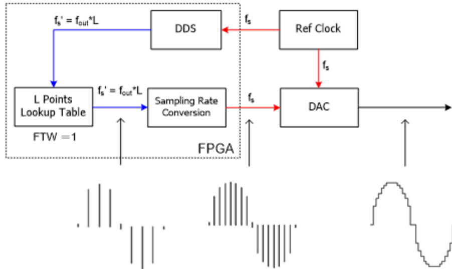
图 12.1 TrueArb 技术原理框图
