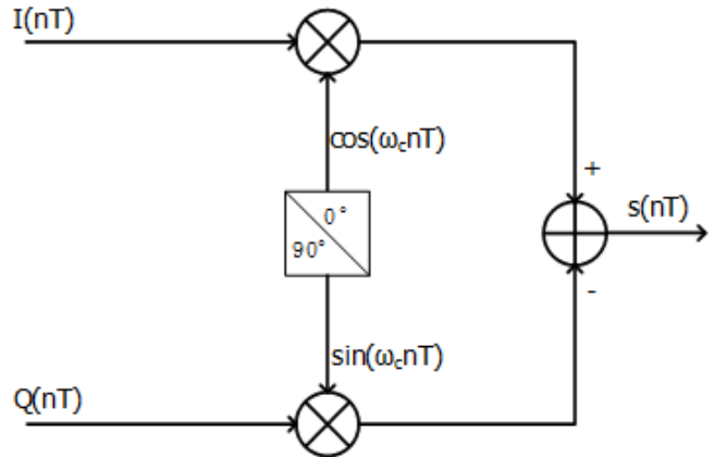
图 13.3 正交调制器的原理框图
