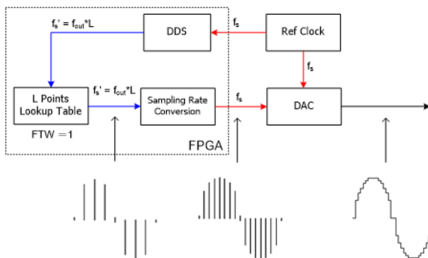
图 10.1 TrueArb 技术原理框图
