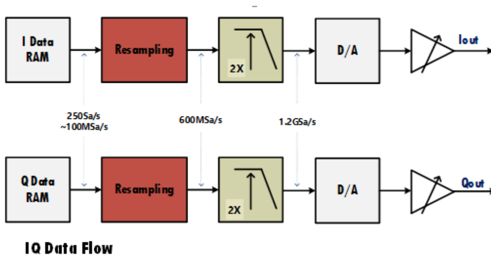
图 11.1 基带 IQ 模式
