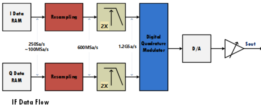
图 11.2 中频信号模式
