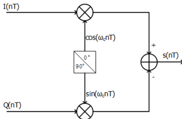
图 11.3 正交调制器的原理框图
