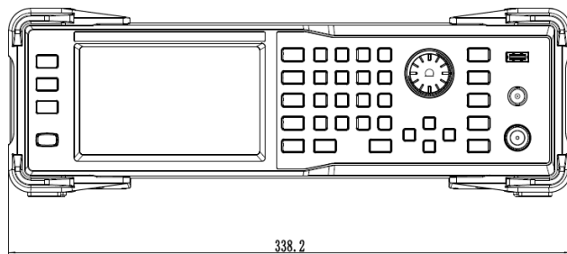
正视图
