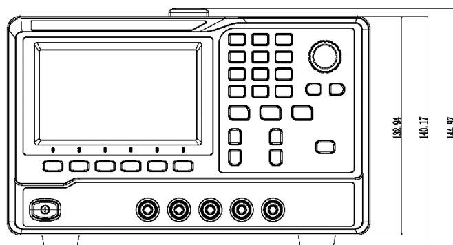
正视图
