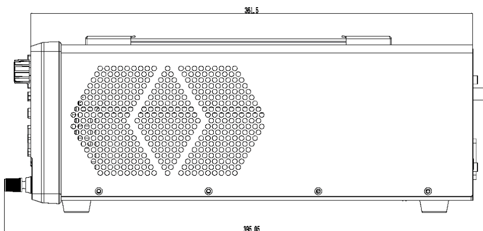
右视图
