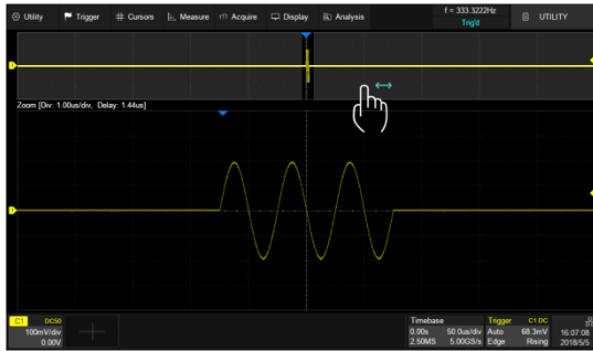
在主波形区的灰色区域左右滑动来控制波形的水平位移
