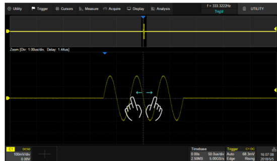
在主波形区的放大区域或 Zoom 波形区通过水平方向的两点缩放手势控制 Zoom 波形区的水平档位
