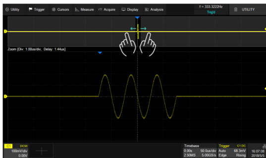
在主波形区的灰色区域通过水平方向的两点缩放手势控制主波形区的水平档位
