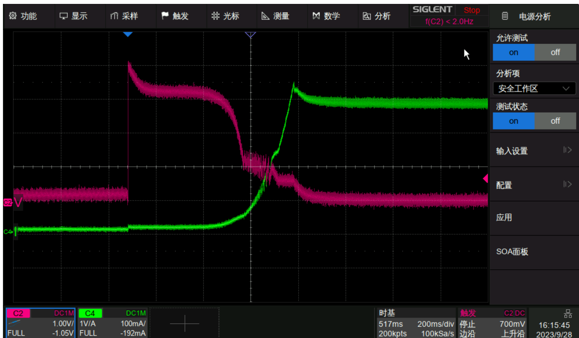
上电时 MOSFET 上的电压和电流波形
