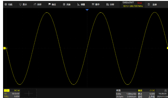
Sinc 插值
