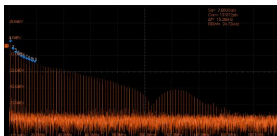
频谱仪模式
