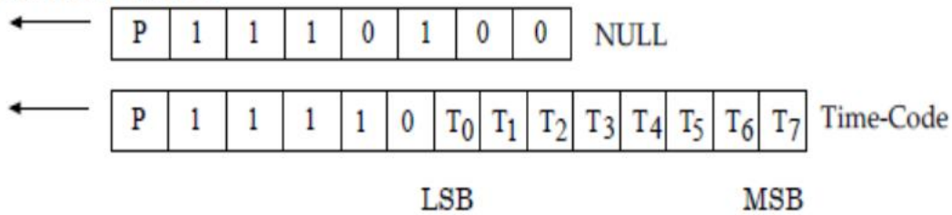
控制码格式
