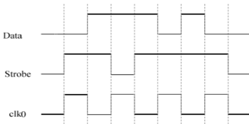
DS 编码和时钟恢复
