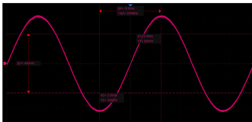
手动模式
