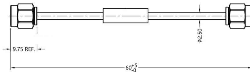
双 SMA 公头线缆
