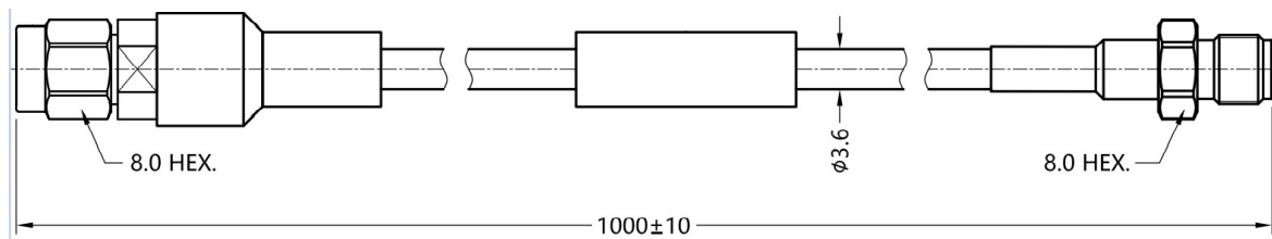
主线缆
