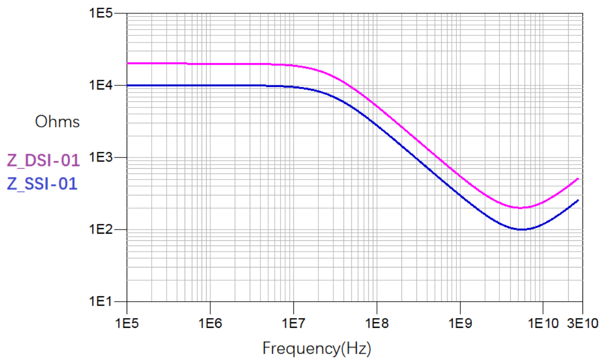
DSI-01 和 SSI-01 的输入阻抗曲线
