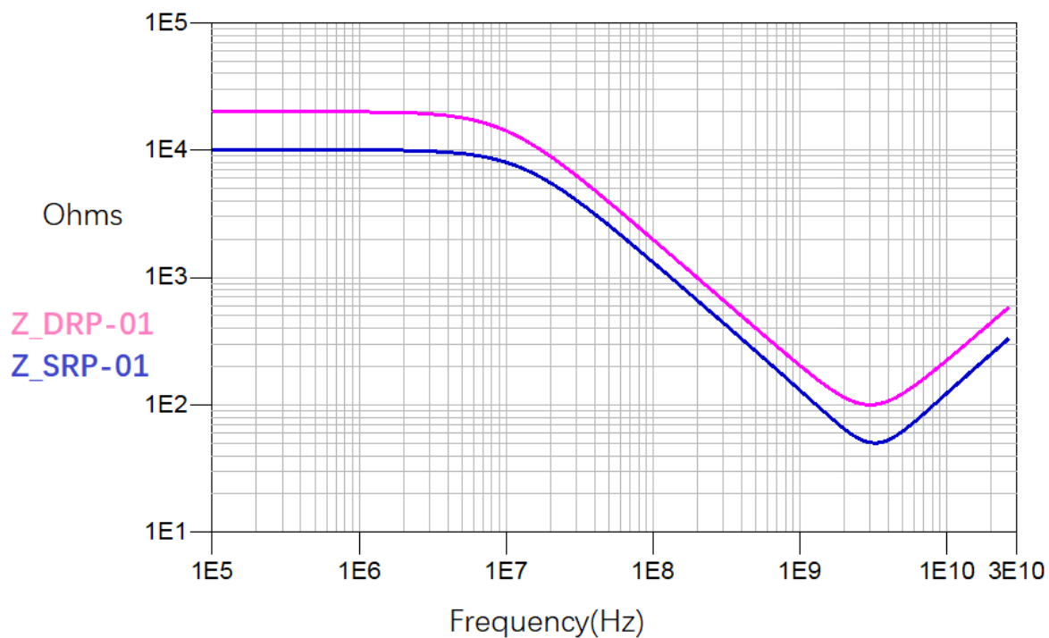
DRP-01 和 SRP-01 的输入阻抗曲线
