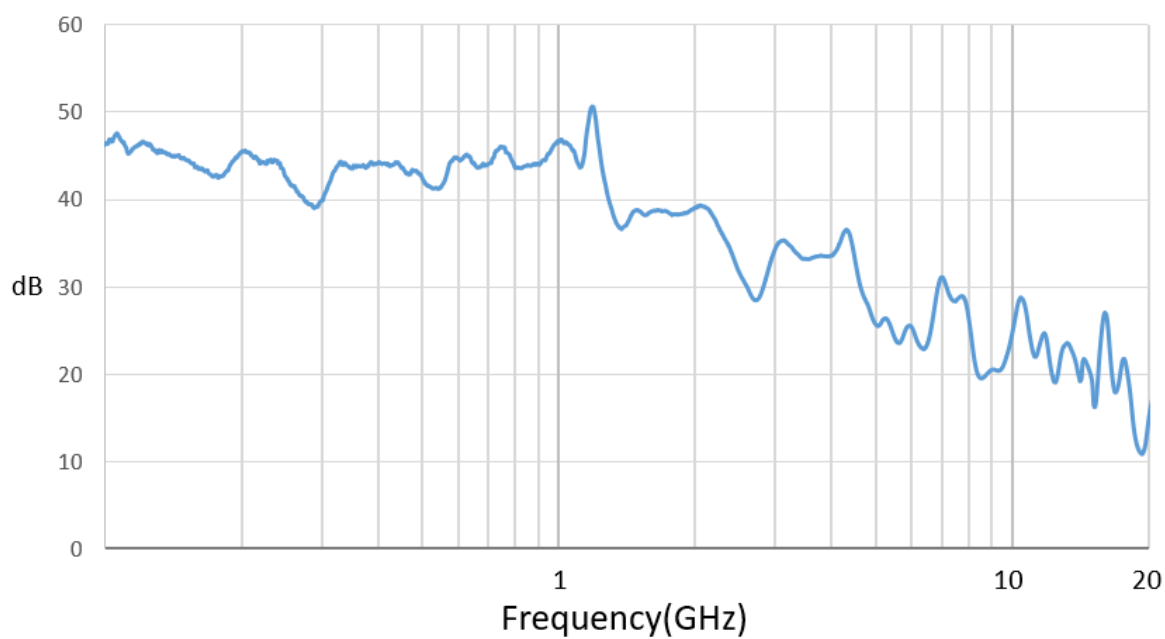
DRP-01 共模抑制比
