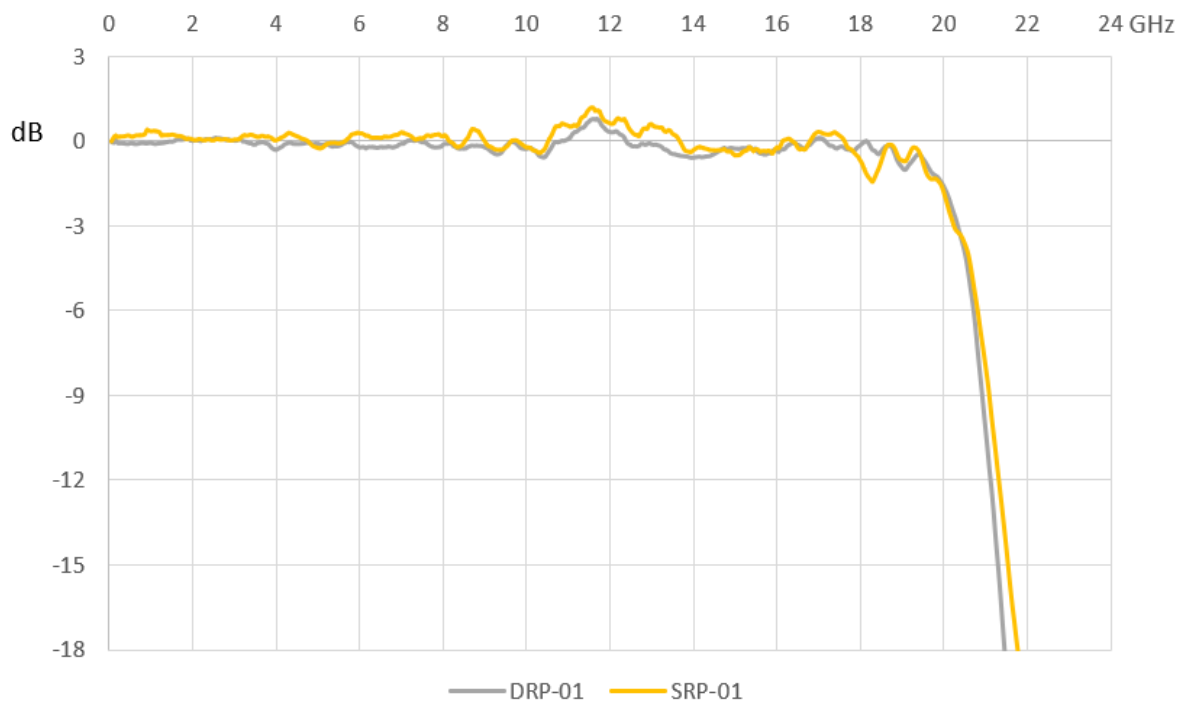
幅频响应曲线 (SAP200D 配合 SDS8204A)
