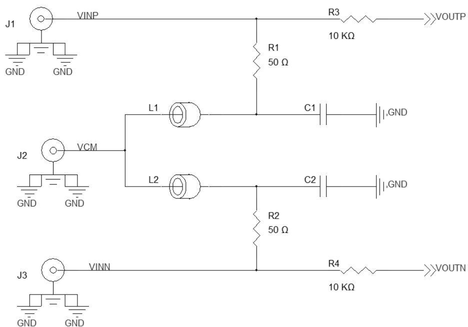
SMA-01 原理简图
