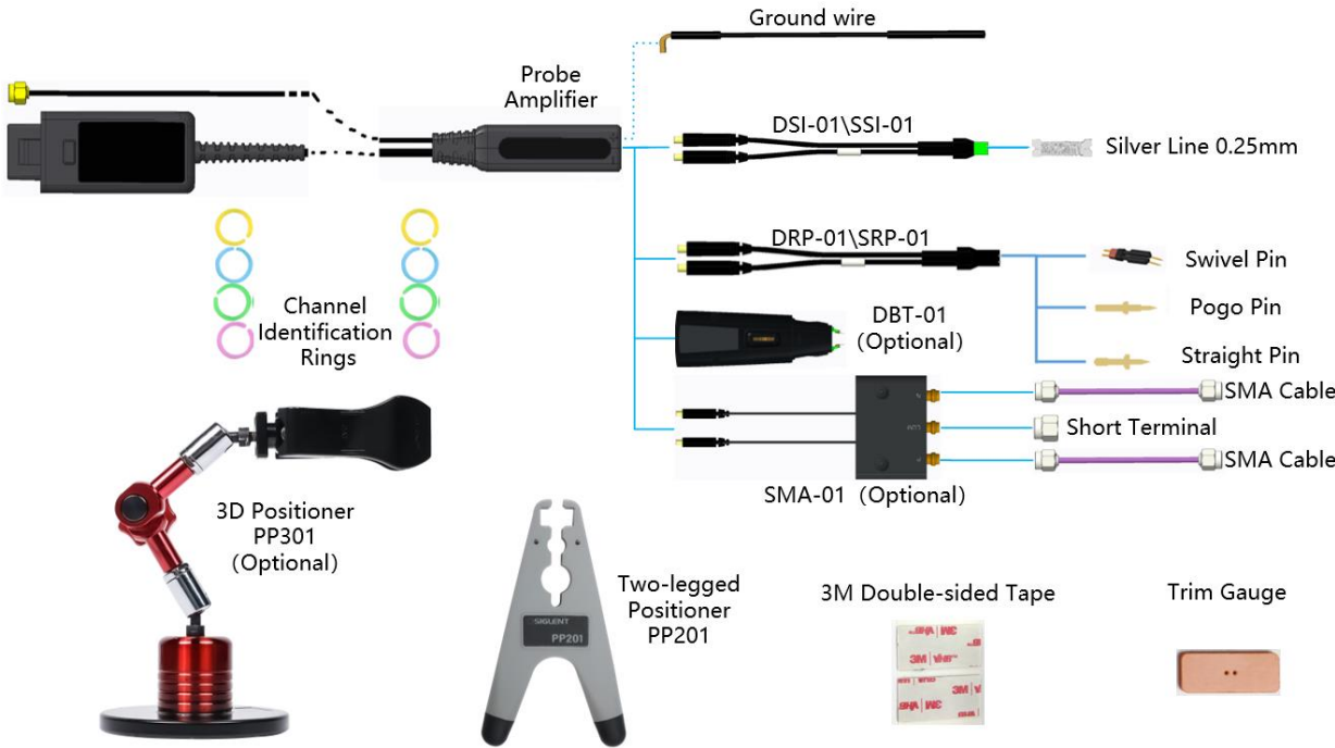
探头配件示意图
