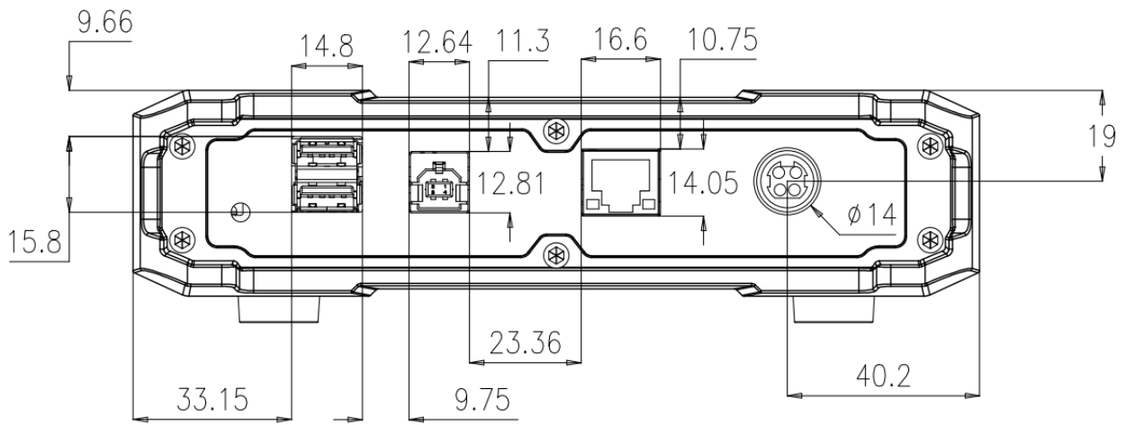
背视图
