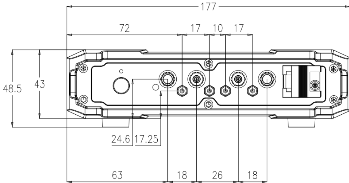
正视图
