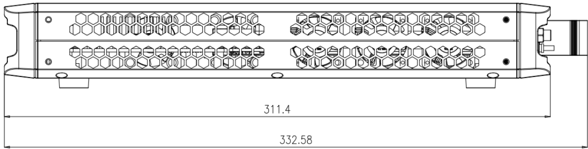
侧视图
