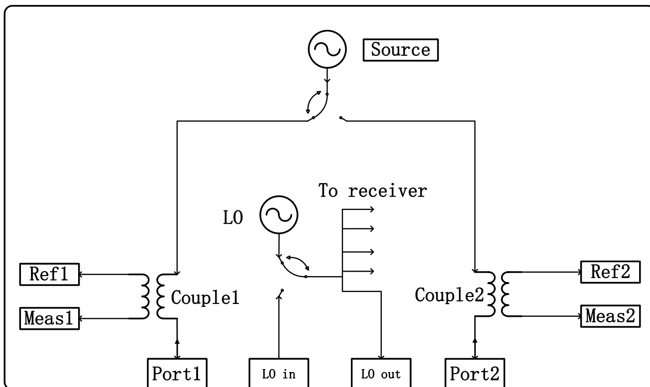
射频示意图
