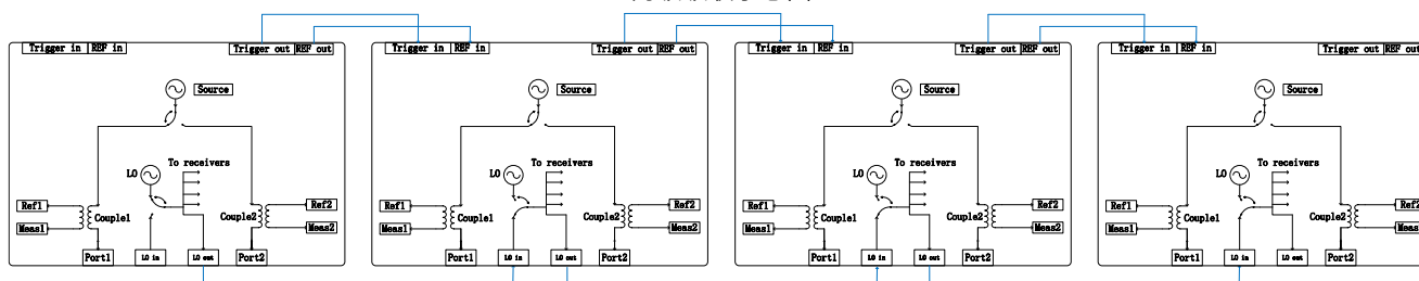
多级级联示意图
