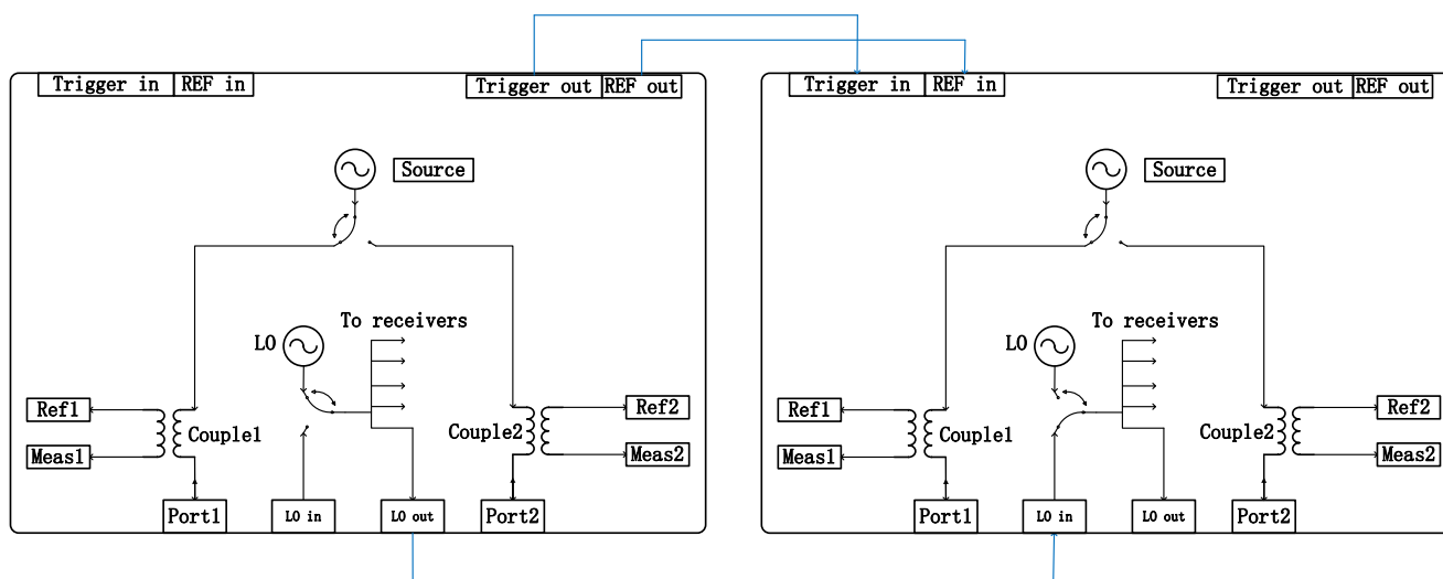
两级级联示意图
