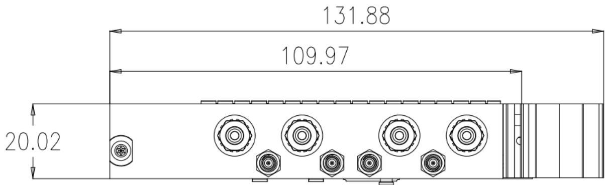
顶视图
